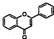
FLAVONE
